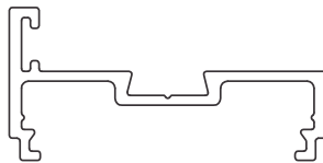
45.04 Door Stop
